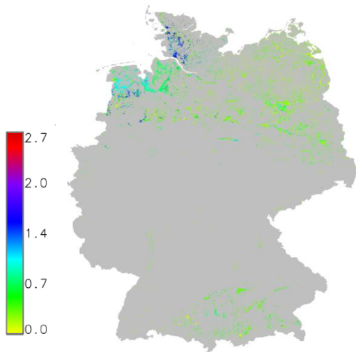
Fig.: Regionalisierte THG Emissionen oranischer Böden a) CO 2 [g CO 2 C m -2 a -1 ]; b) N 2 O [N 2 O N ha -2 a -1 ]
